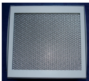
Das Alu-Drahtgewirrfilter entspricht der Filterklasse G2 (DIN EN 779/ 2002).
