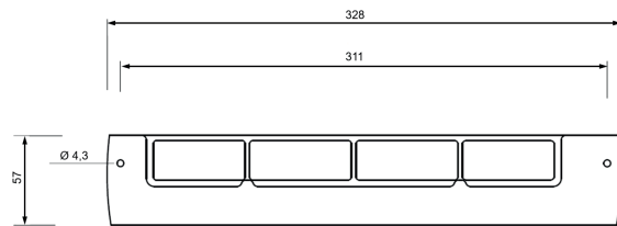
Gittergrundplatte ROIS 02 - Frontansicht
